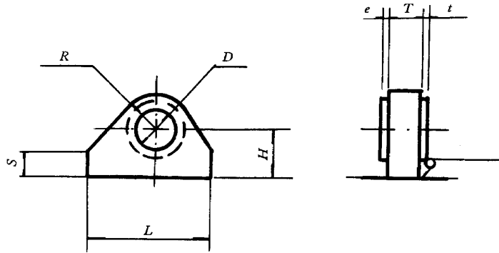
图 C1 吊耳
